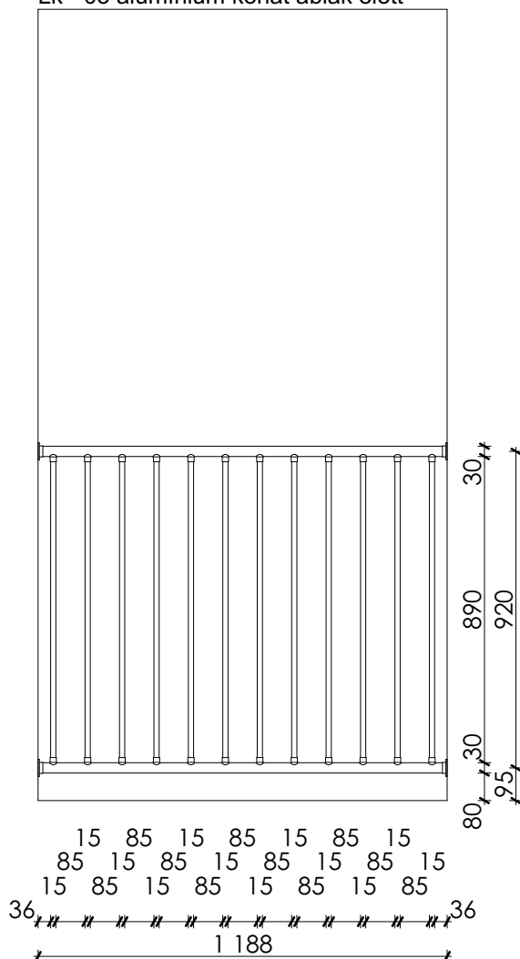
Lk - 03 alumínium korlát ablak előtt
